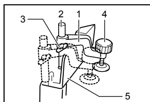
1. Bras de l'étau 2. Tige de l'étau 3. Vis 4. Bouton de l'étau 5. Garde de guidage
