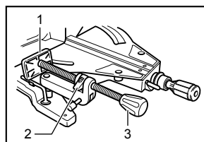
1. Plaque de l'étau 2. Écrou de l'étau 3. Bouton de l'étau
