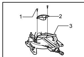
1. Vis 2. Bloc de découpe 3. Garde de guidage
