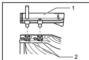
1. Garde auxiliaire de droite 2. Vis
