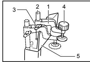
1. Brazo de la mordaza 2. Barra de la mordaza 3. Tornillo 4. Perilla de la mordaza 5. Guía lateral
